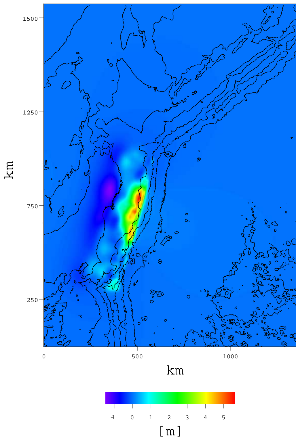
図. 初期水位分布
